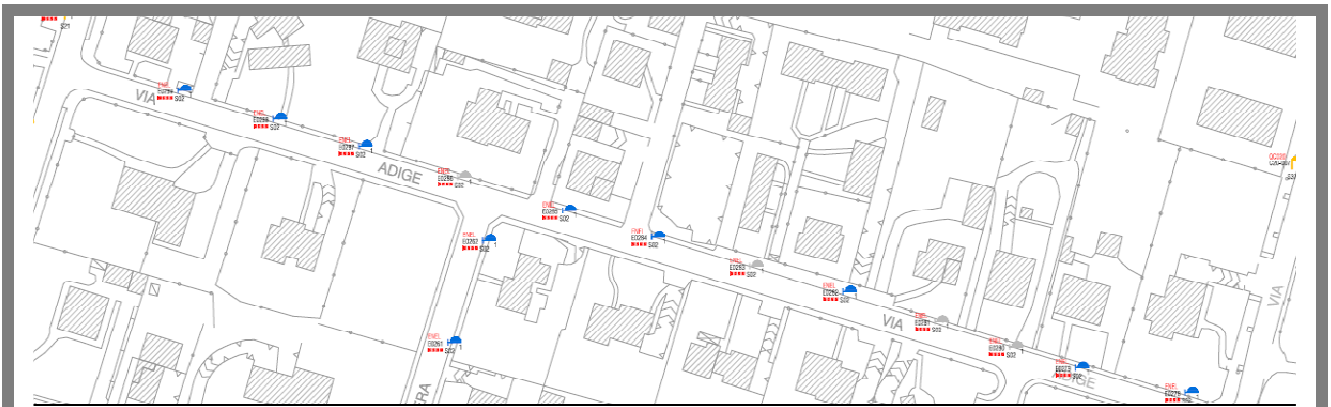
Censimento dei dispositivi illuminanti Via Adige
